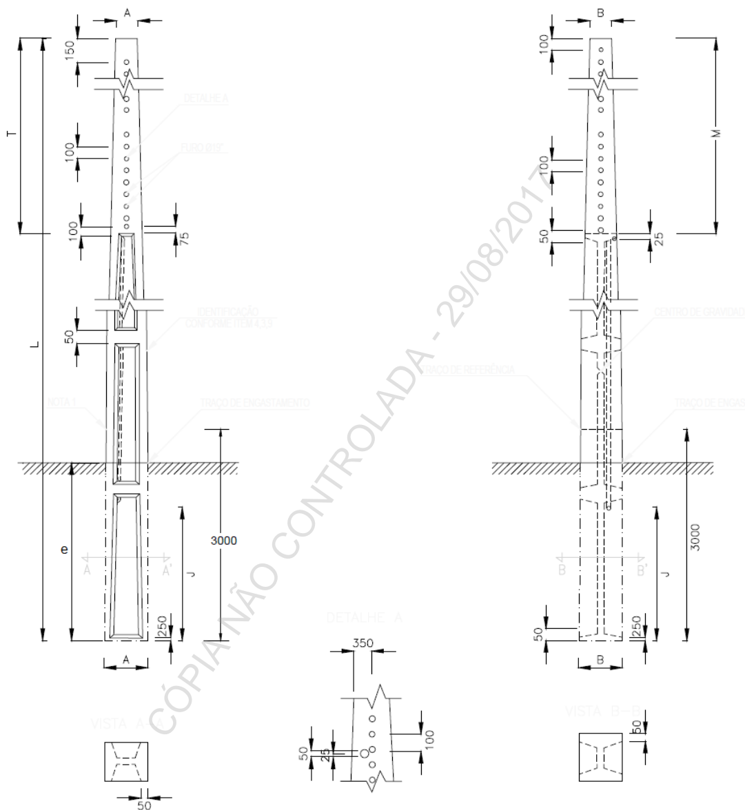
Figura 1 - Postes de Concreto Seção Duplo T – Distribuição
