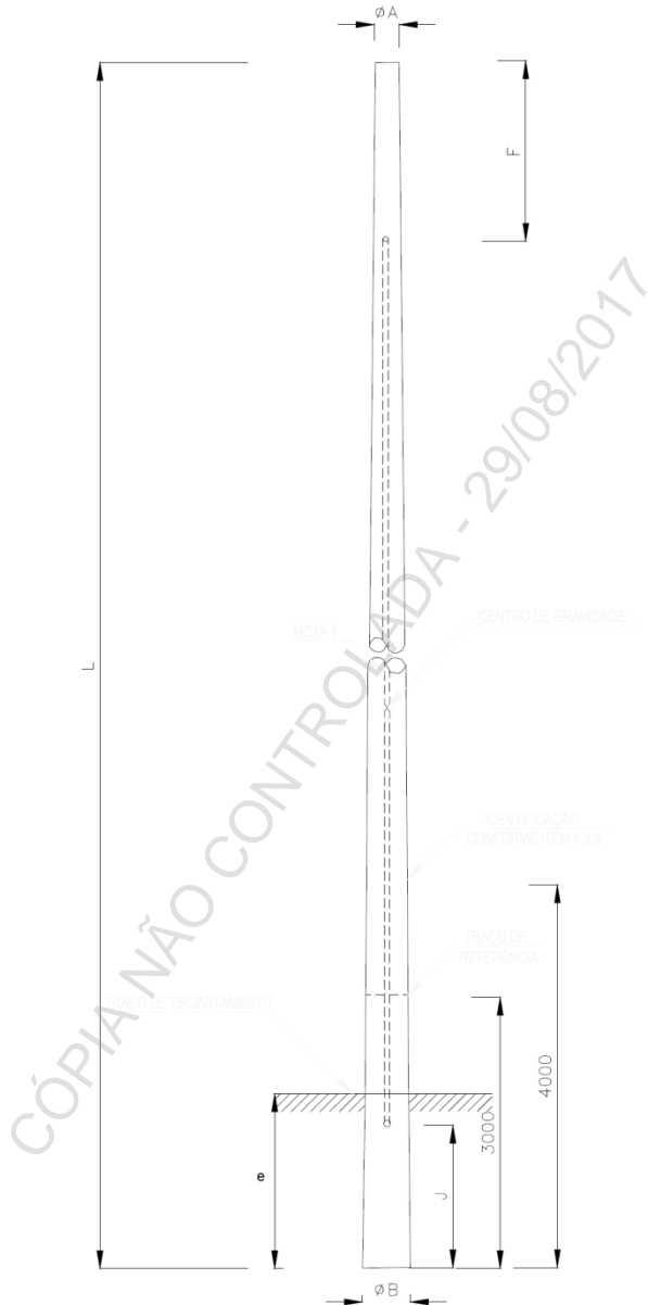
Figura 2 - Postes de Concreto Seção Circular (C) - Distribuição
