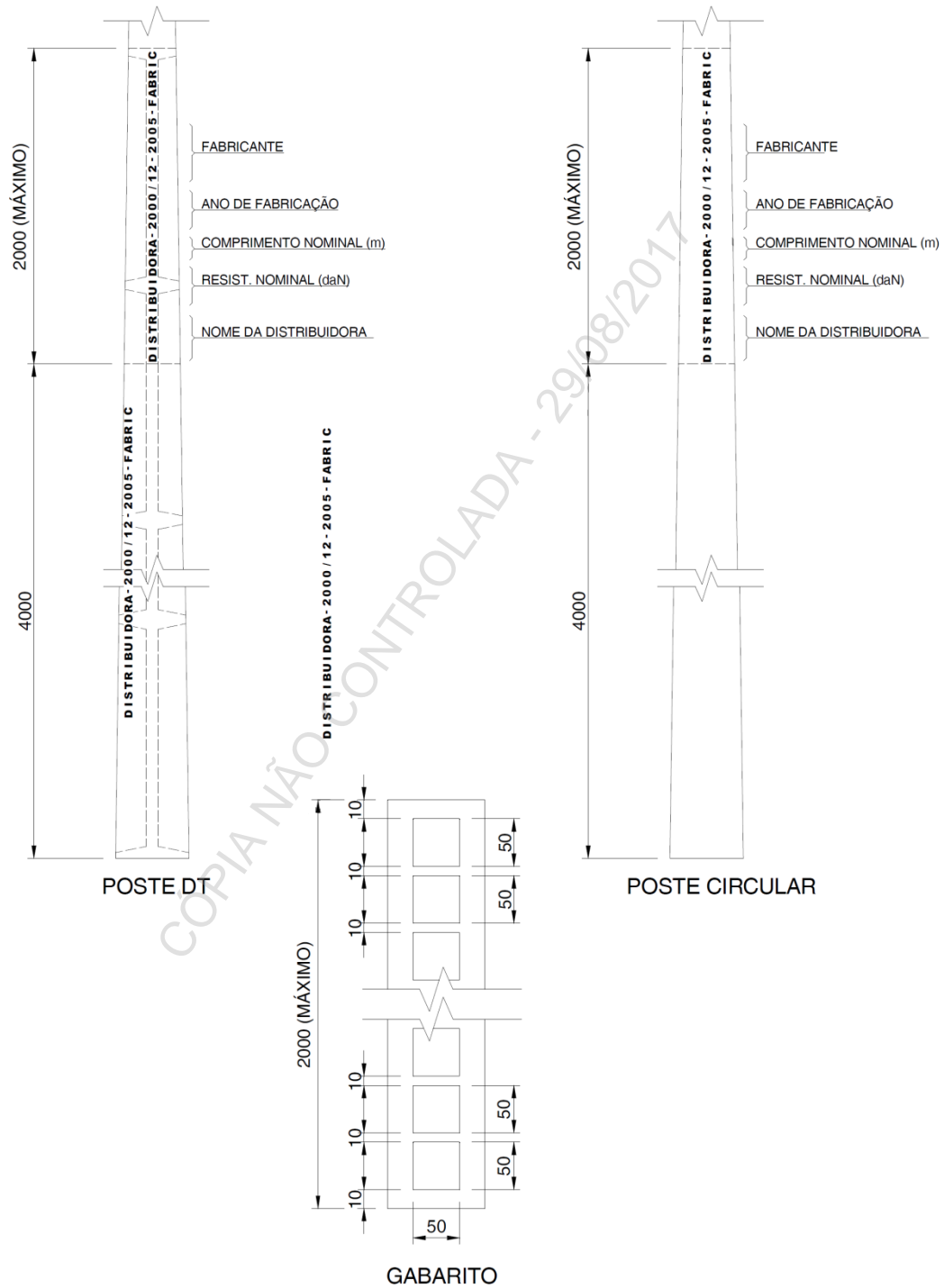
Figura 3 - Identificação do Poste - Distribuição
