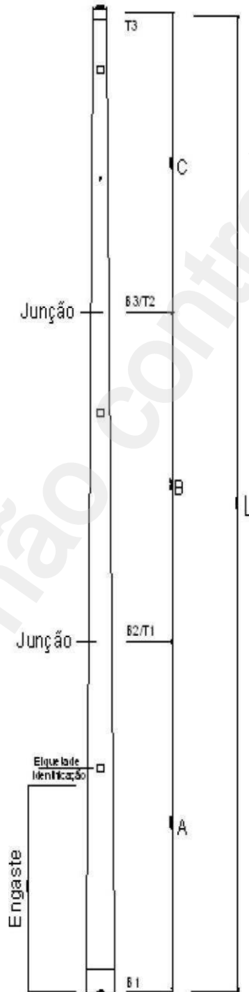
Figura 3 - Poste de Fibra Seccionável (Topo e Base Circulares)
